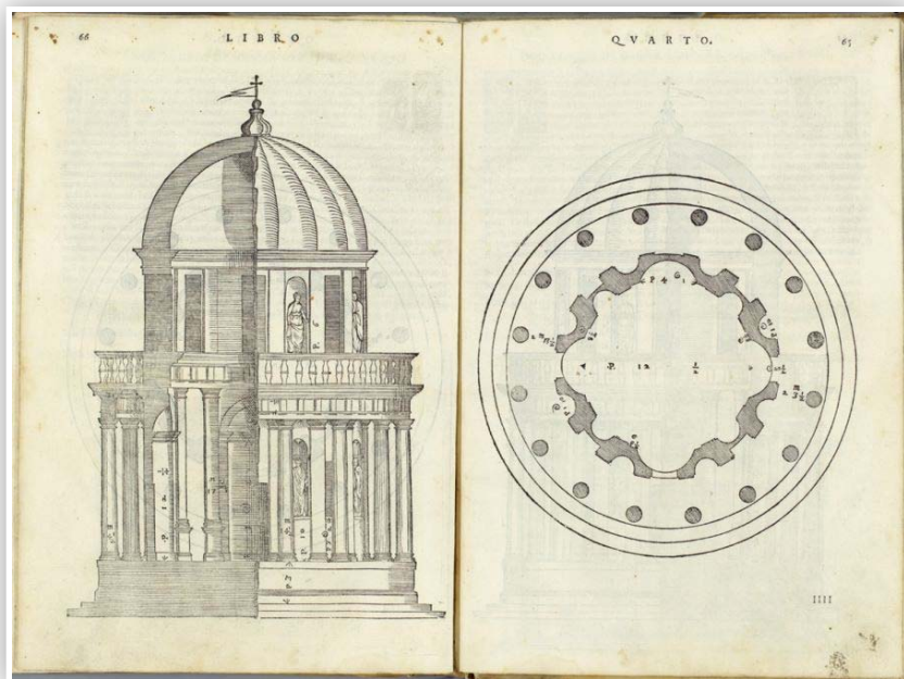
Prospetto, sezione del tempio di Bramante in Andrea Palladio, I Quattro libri dell'architettura di Andrea Palladio, Venezia, 1570, libro IV,
